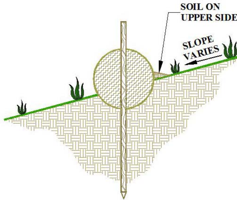
ENTRENCHMENT DETAIL N.T.S.
