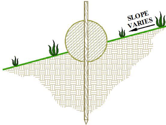
ENTRENCHMENT DETAIL N.T.S.
